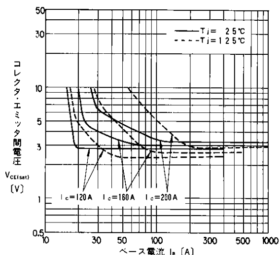
出力特性
