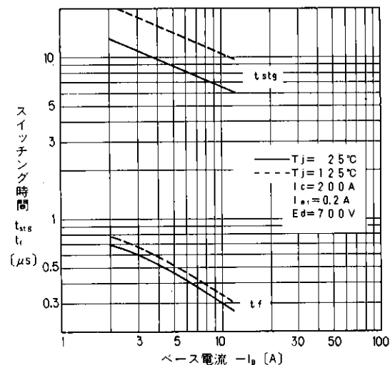
スイッチング時間—ベース電流特性
