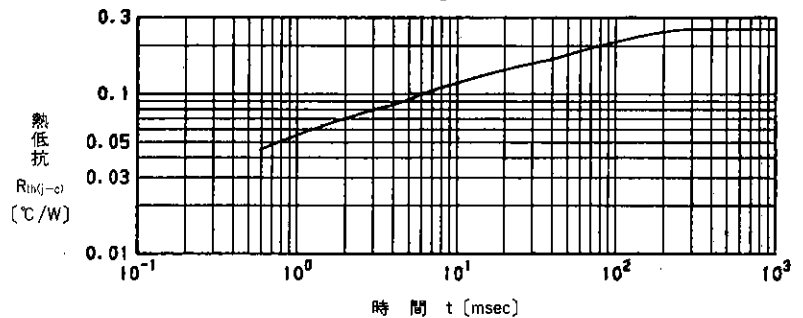
過渡熱抵抗(トランジスタ)特性 Transient Thermal Resistance (Transistor)
