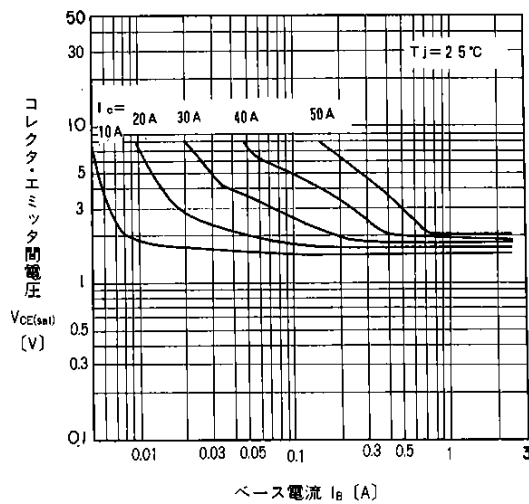
出力特性
