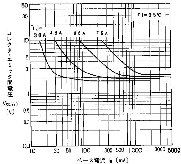
出力特性
