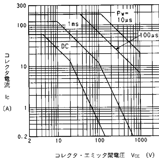
コレクタ・エミッタ間電圧 V_{CE} (V) 安全動作領域特性
