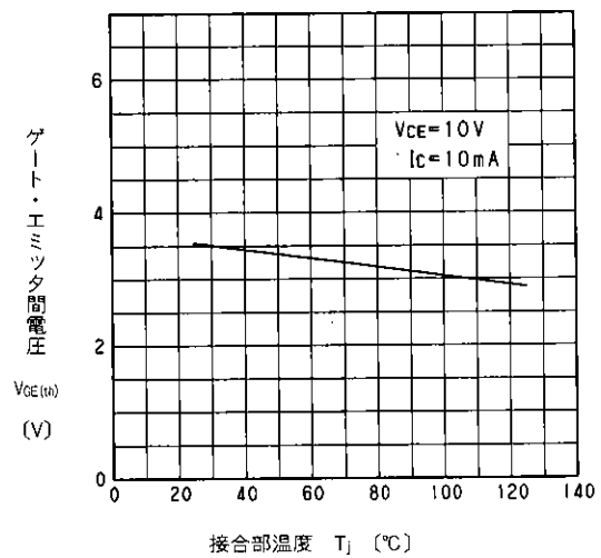
ゲートしきい値電圧-接合部温度特性(標準値)
