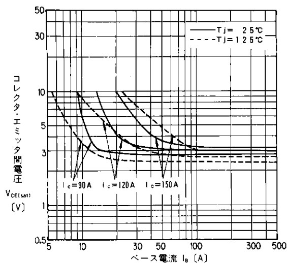
出力特性
