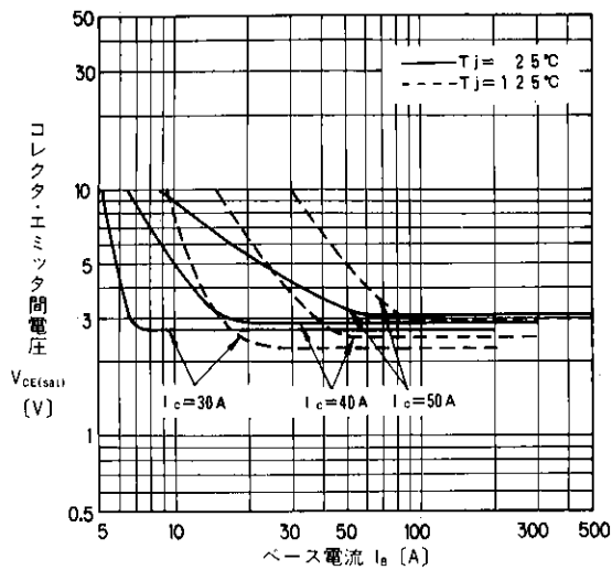
出力特性
