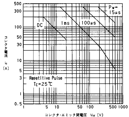
安全動作領域 (繰返し) Safe Operating Area
