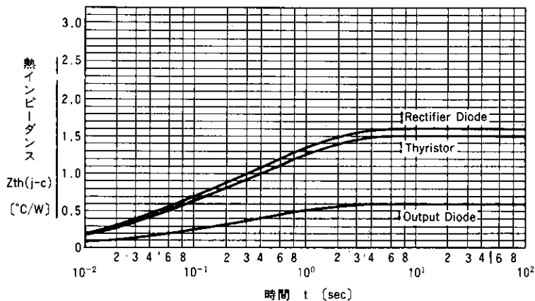
過渡熱インピーダンス(1素子あたり, 接合—ケース間) Transient Thermal Impedance (per 1 chip, Junction to Case)
