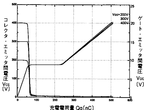
充電電荷量 Q_g (nC) ダイナミック入力特性 ( T_j = 25^\circ\text{C} ) <INV部> Dynamic input characteristic <INV>
