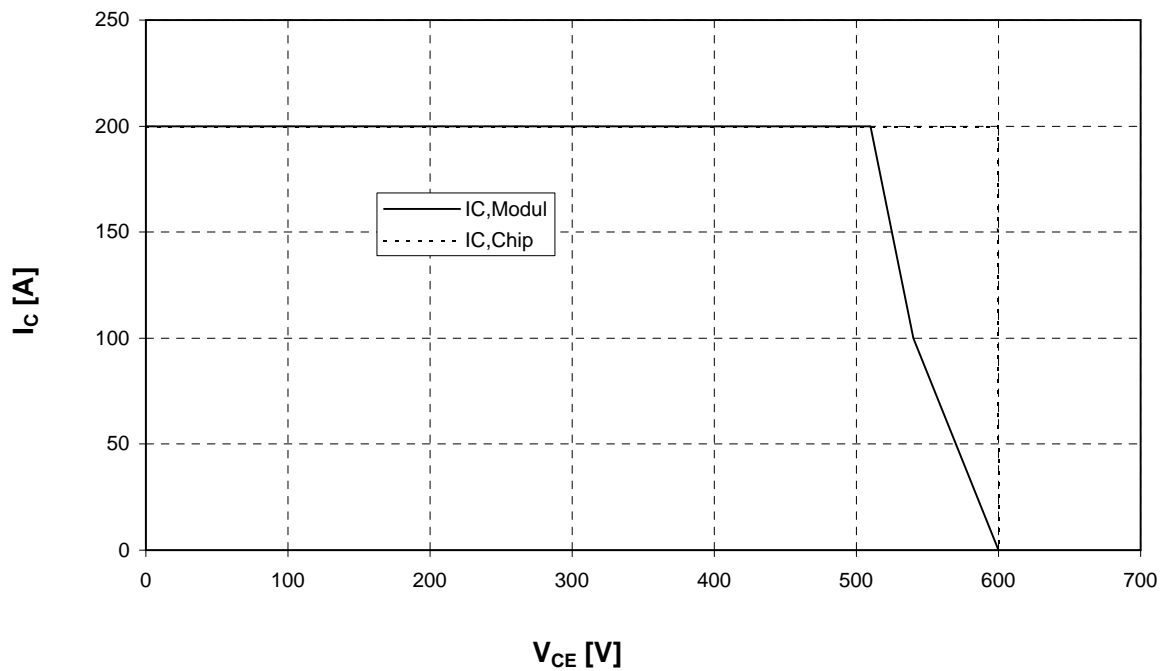
Sicherer Arbeitsbereich Wechselr. (RBSOA) I_c = f(V_{CE}) Reverse bias safe operating area Inverter (RBSOA) T_{vj} = 125^\circ\text{C}, V_{GE} = \pm 15\text{V}, R_G = 15 \text{ Ohm}
