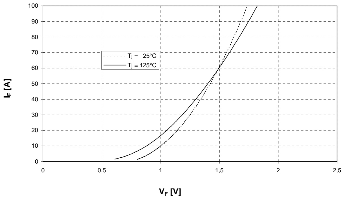
Durchlaßkennlinie der Brems-Chopper-Diode (typisch) i = f(V_F) Forward characteristic of brake-chopper-FWD (typical)
