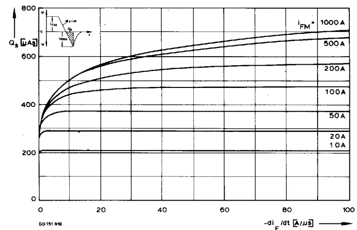
Bild/Fig. 6 Nachlaufladung Q_S in Abhängigkeit von der abkommutierenden Stromsteilheit -di_F/dt bei t_{vj \max} . Lag charge Q_S versus the rate of decay of the forward current -di_F/dt at t_{vj \max} .
