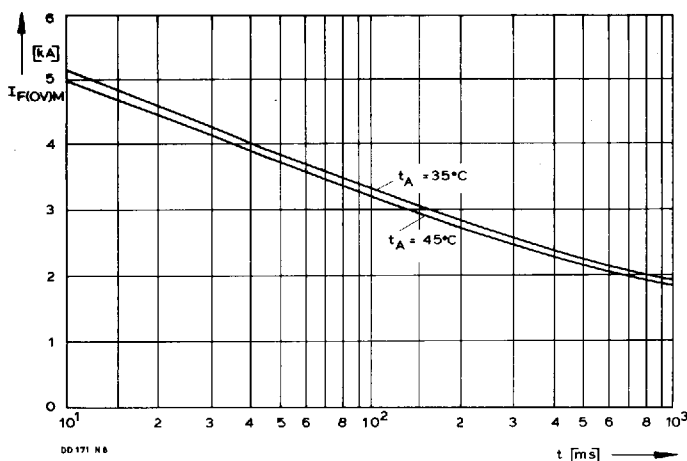
Bild/Fig. 5 Grenzstrom je Zweig I_{FOVIM} bei Luftselbstkühlung, t_A = 45^\circ\text{C} und verstärkter Luftkühlung, t_A = 35^\circ\text{C} , Belastung nach Leerlauf, v_{RM} = 0.8 V_{RRM} . Limiting overload on-state current per arm I_{FOVIM} at natural ( t_A = 45^\circ\text{C} ) and forced ( t_A = 35^\circ\text{C} ) cooling, current surge under no-load conditions, v_{RM} = 0.8 V_{RRM} .
