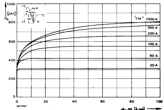
Bild/Fig. 6 Nachlaufladung Q_S in Abhängigkeit von der abkommutierenden Stromsteilheit -di_F/dt bei t_{vj \max} . Lag charge Q_S versus the rate of decay of the forward current -di_F/dt at t_{vj \max} .
