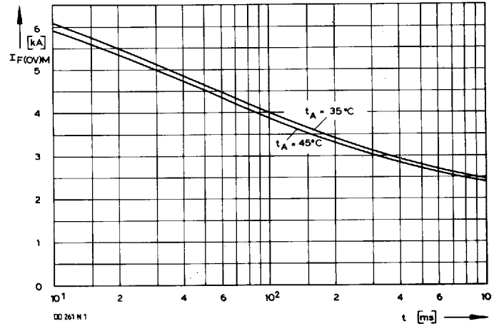
Bild/Fig. 6: DD 261 N Grenzstrom je Zweig I_{F(OV)M} bei Luftselbstkühlung, t_A = 45^\circ\text{C} und verstärkter Luftkühlung, t_A = 35^\circ\text{C} , Belastung nach Leerlauf, V_{RM} = 0.8 V_{RRM} . Limiting overload on-state current per arm I_{F(OV)M} at natural ( t_A = 45^\circ\text{C} ) and forced ( t_A = 35^\circ\text{C} ) cooling, current surge under no-load conditions, V_{RM} = 0.8 V_{RRM} .
