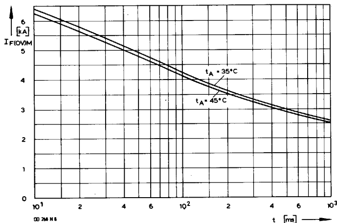
Bild/Fig. 5: DD 260 N Grenzstrom je Zweig I_{F(OV)M} bei Luftselbstkühlung, t_A = 45^\circ\text{C} und verstärkter Luftkühlung, t_A = 35^\circ\text{C} , Belastung nach Leerlauf, V_{RM} = 0.8 V_{RRM} . Limiting overload on-state current per arm I_{F(OV)M} at natural ( t_A = 45^\circ\text{C} ) and forced ( t_A = 35^\circ\text{C} ) cooling, current surge under no-load conditions, V_{RM} = 0.8 V_{RRM} .
