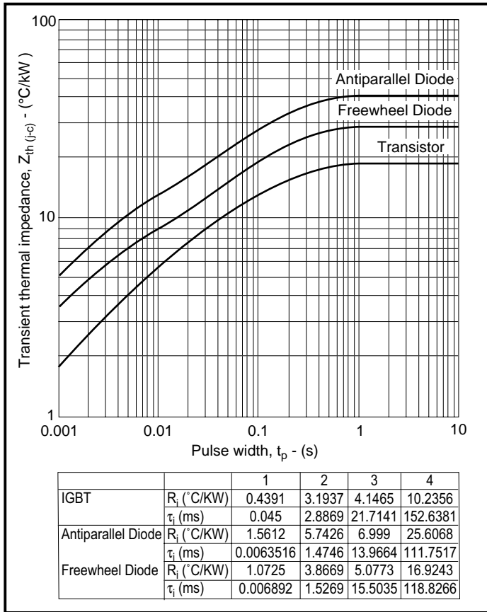
Fig. 13 Transient thermal impedance
