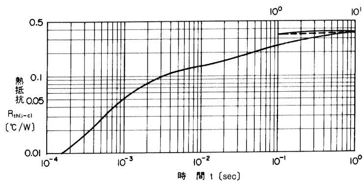
過渡熱抵抗(トランジスタ)特性
