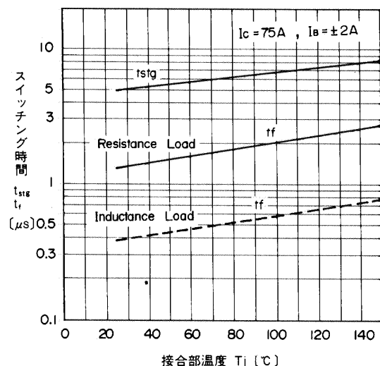
スイッチング時間-接合温度特性
