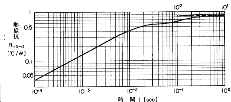
過渡熱抵抗(ダイオード)特性
