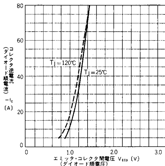
高速フリーホイリングダイオード順電圧 Forward Voltage of Free Wheeling Diode *Switching Time Test Circuit
