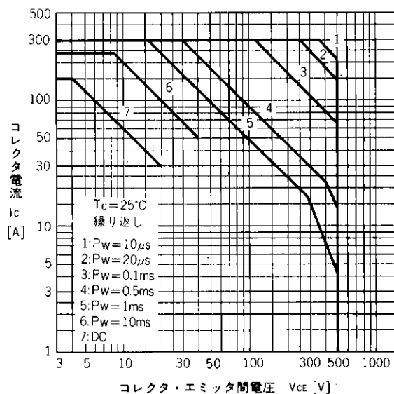
安全動作領域特性(繰り返し) Safe Operating Area
