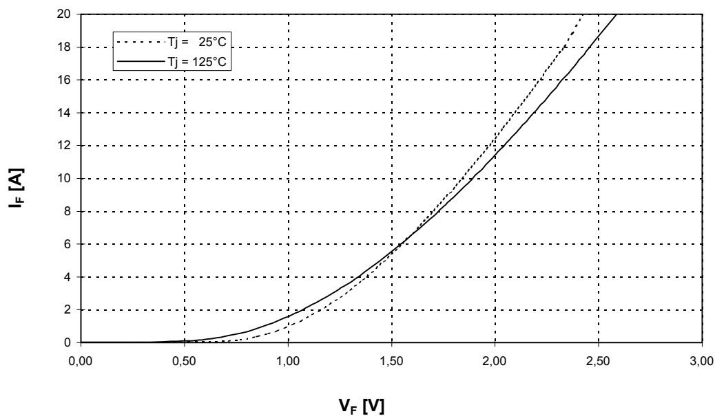
Durchlaßkennlinie der Freilaufdiode Wechsellr. (typisch) I_F = f(V_F) Forward characteristic of FWD Inverter (typical)
