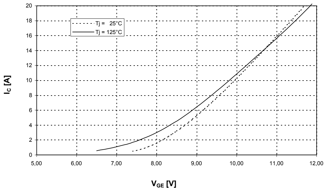
Übertragungscharakteristik Wechsellr. (typisch) Transfer characteristic Inverter (typical)
