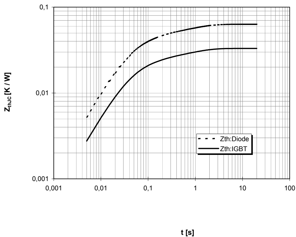
Transienter Wärmewiderstand Transient thermal impedance
