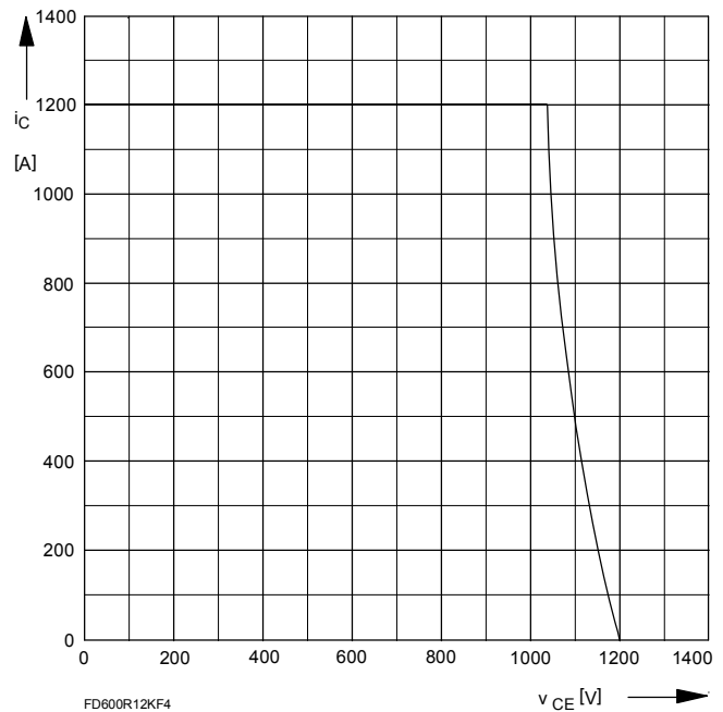
Bild/Fig. 4 Rückwärts-Arbeitsbereich Reverse biased safe operating area t_{vj} = 125\text{ °C} , v_{LF} = v_{LR} = 15V , R_G = 1,6W
