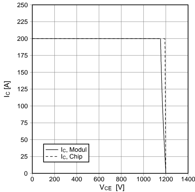
Sicherer Rückwärts-Arbeitsbereich IGBT-Wr. (RBSOA) reverse bias safe operating area IGBT-inv. (RBSOA) I_C = f(V_{CE}) V_{GE} = \pm 15\text{ V} , R_{Goff} = 9,1\ \Omega , T_{vj} = 125^\circ\text{C}
