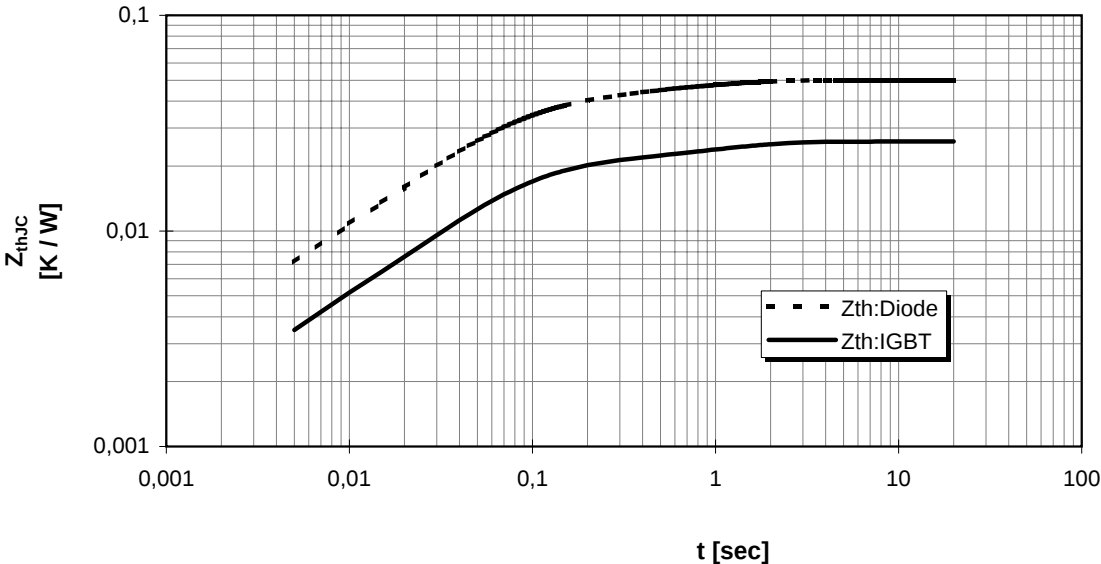
Transienter Wärmewiderstand Transient thermal impedance
