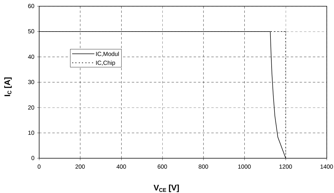
Sicherer Arbeitsbereich IGBT-Wechsele. (RBSOA) Reverse bias safe operating area (RBSOA)
