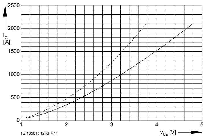
Bild / Fig. 1 Kollektor-Emitter-Spannung im Sättigungsbereich (typisch) / Collector-emitter-voltage in saturation region (typical) V_{GE} = 15\text{ V} ----- T_{vj} = 25^\circ\text{C} ———— T_{vj} = 125^\circ\text{C}
