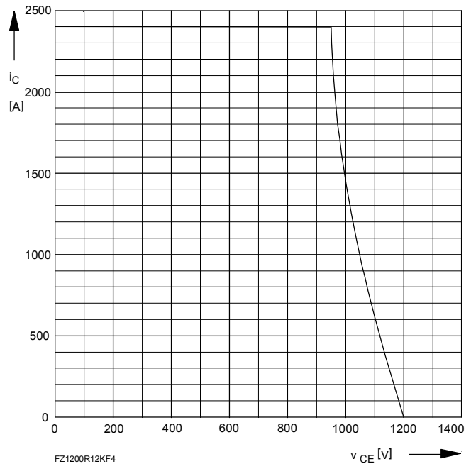
Bild/Fig. 4 Rückwärts-Arbeitsbereich Reverse biased safe operating area t_{vj} = 125\text{ °C} , v_{LF} = v_{LR} = 15\text{ V} , R_G = 0,82\Omega
