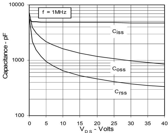
Fig. 11. Capacitance
