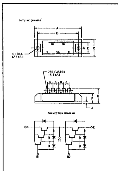
1200 Volt KD7212A2 Outline Drawing
