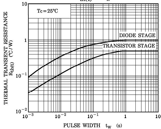
R_{th}(t) - t_w
