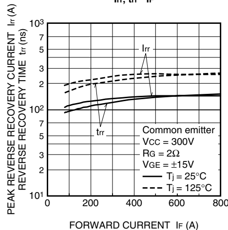
I_{rr} , t_{rr} - I_F
