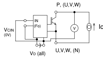
Fig. 1 V_{CE(sat)} Test
