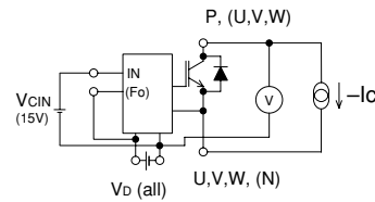
Fig. 2 V_{EC} Test
