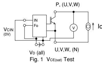
Fig. 1 V_{CE(sat)} Test
