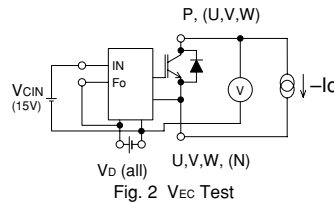
Fig. 2 V_{EC} Test
