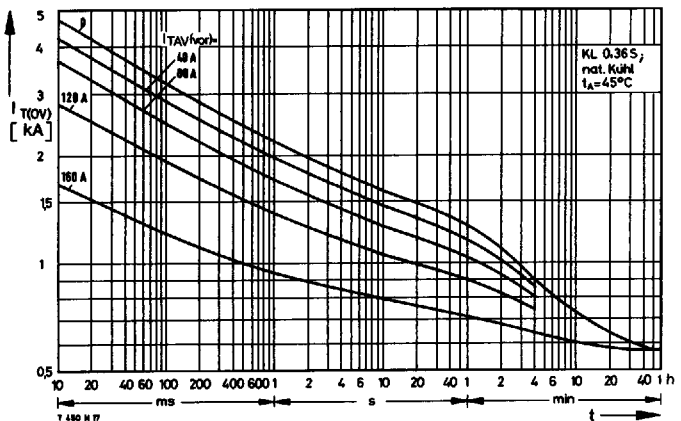
Bild/Fig. 14 Überstrom I_{T(ON)} bei beidseitiger Luftselbstkühlung, t_A = 45^{\circ}\text{C} , Kühlkörper K0.36 S. Overload on-state current I_{T(ON)} at natural two-sided cooling, t_A = 45^{\circ}\text{C} , heatsink type K0.36 S. Parameter: Vorlaststrom/pre-load current I_{TAV(vor)}
