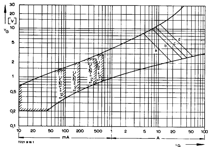
Bild/Fig. 19 Zündbereich und Spitzensteuerleistung bei v_D \geq 6 \text{ V} . Gate characteristic and peak gate power dissipation at v_D \geq 6 \text{ V} . Parameter: a b c d Steuerimpulsdauer/Pulse duration t_g [ms] 10 1 0,5 0,1 Höchstzulässige Spitzensteuerleistung/Maximum allowable peak gate power [W] 40 80 100 150
